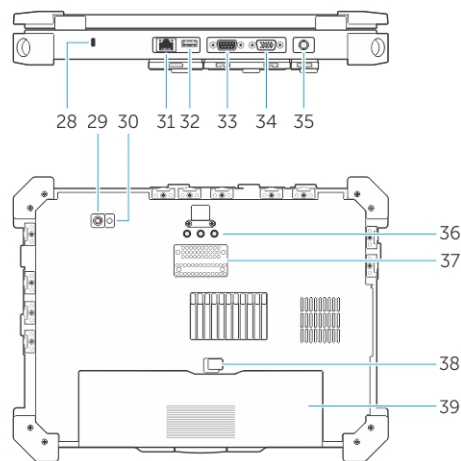
Abbildung 1. Systemübersicht
