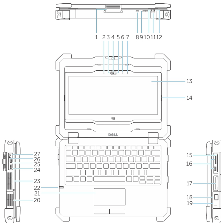
Afbeelding 1. Systemoverzicht
